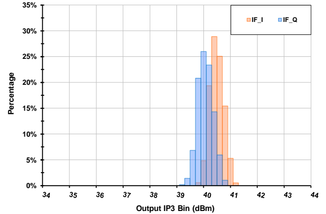
Output IP3 (N = 2724)
