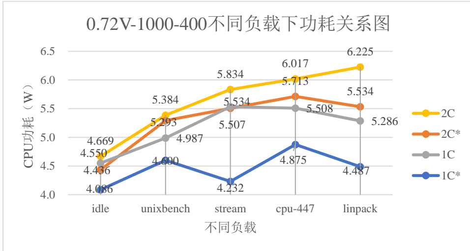
图 6.1 0.72V-1000-400 不同负载下功耗关系图
