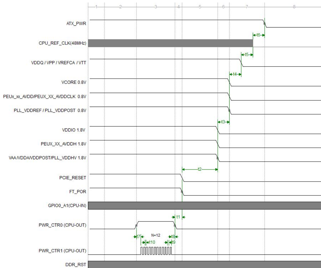
图 5.2 S0→S4/S5 关机时序图
