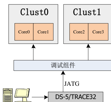
图 2.21 FT-2000/4 软件调试结构
