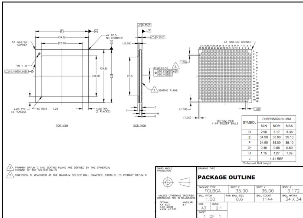
图 8.1 封装机械尺寸
