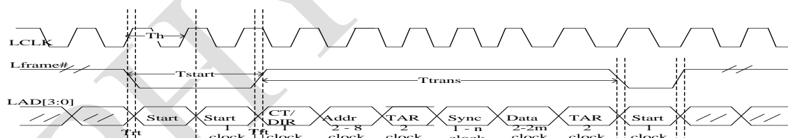
图 2.3 GMAC 开关特性图
