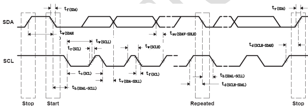
图 2.11 I2C 发送时序
