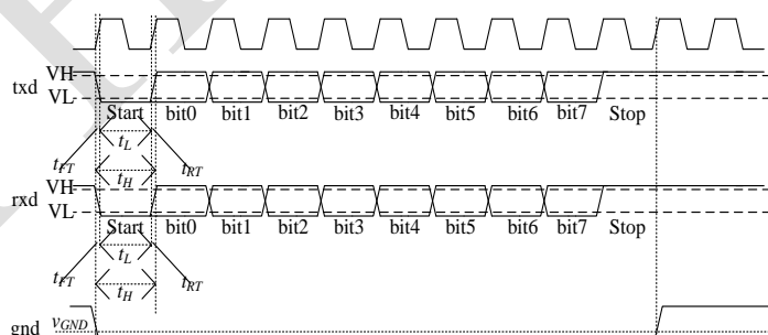
图 2.16 UART 时序图
