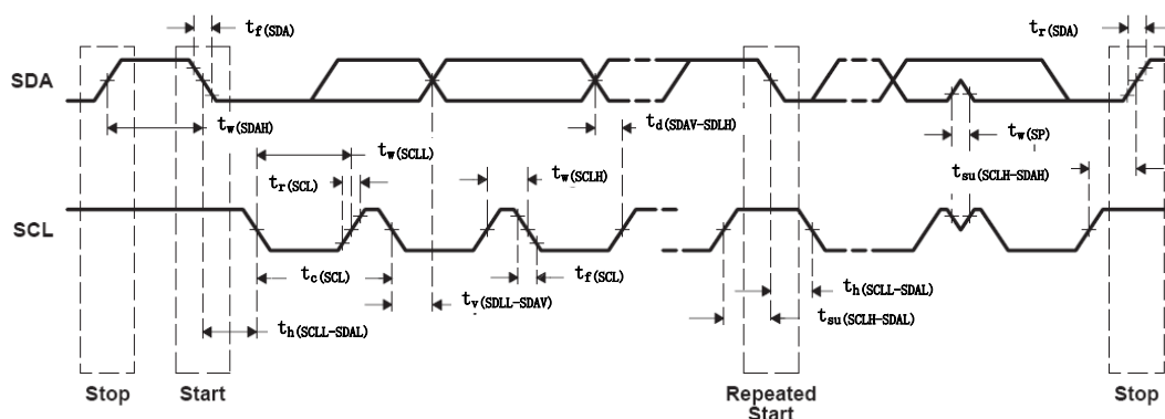
图 2.10 I2C 接收时序
