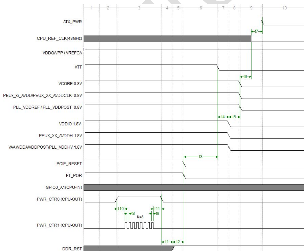
图 5.3 S0→S3 休眠时序图
