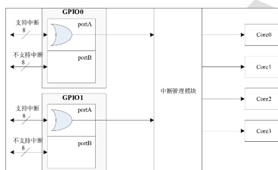
图 2.17 GPIO 中断结构图
