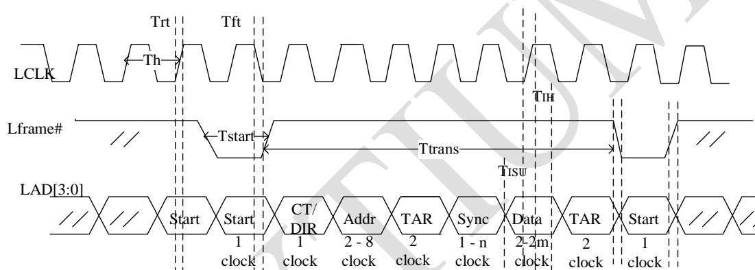
图 2.15 LPC 基本时序
