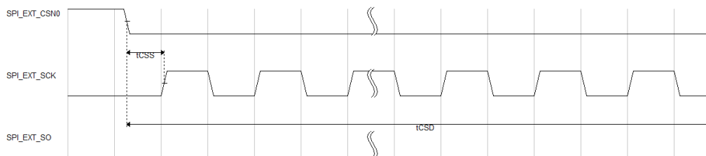
图 2.14 SPI 时序图
