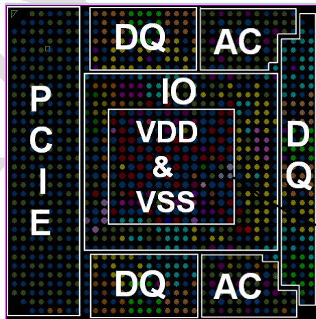
图 8.3 BGA MAP 分布图
