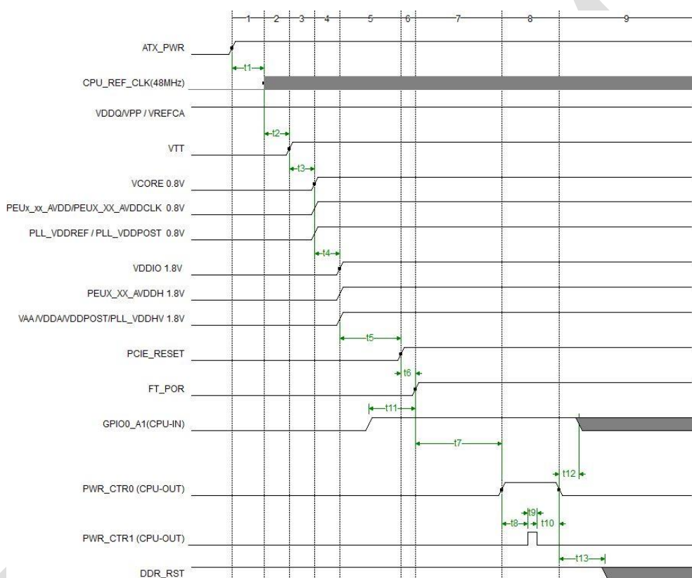
图 5.5 S3→S0 唤醒时序图
