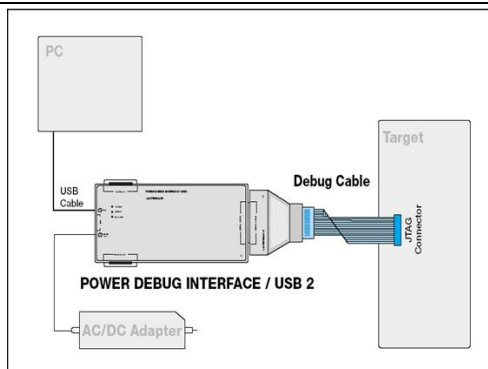
图 2.22 trace32 连接 PC 进行调试
