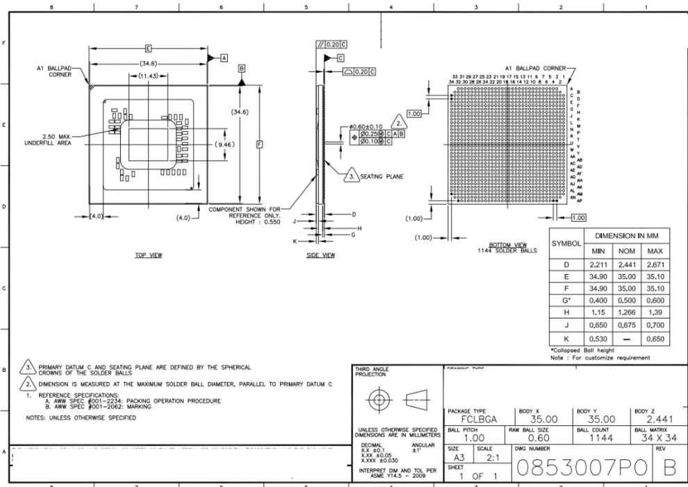
图 8.2 FT-2000/4 移动版封装机械尺寸
