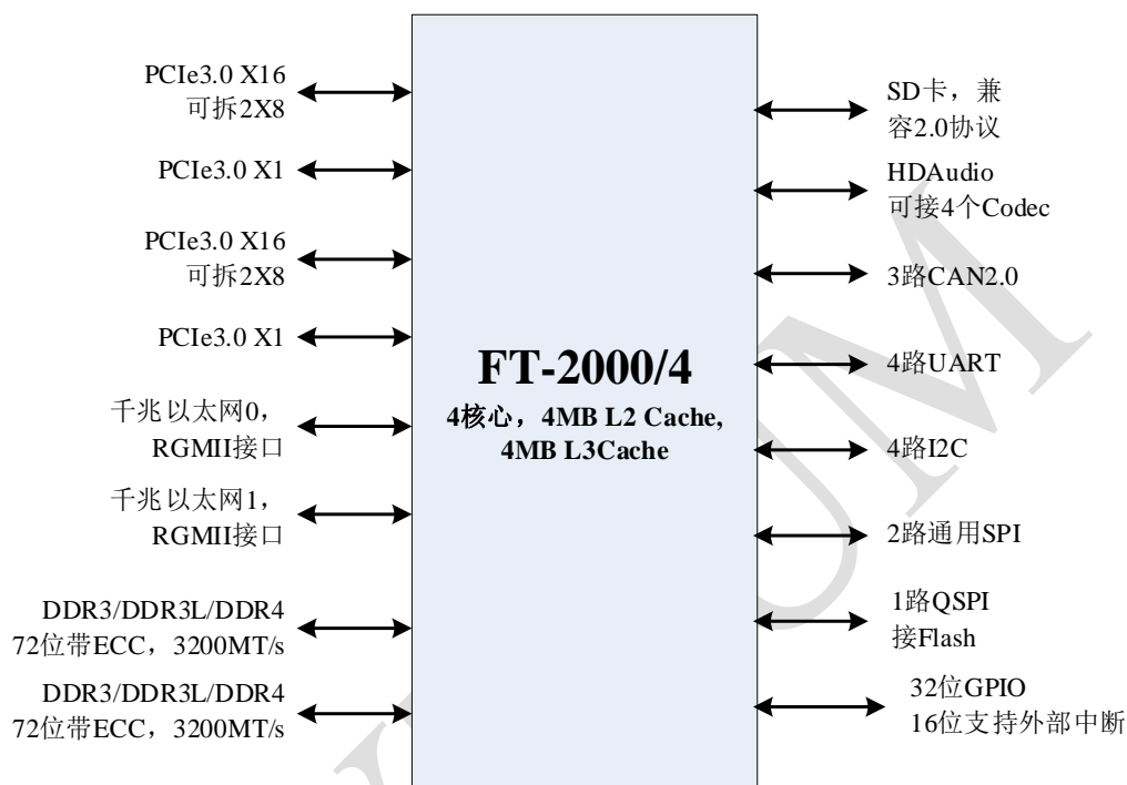
图 2.1 FT-2000/4 处理器接口信号框图
