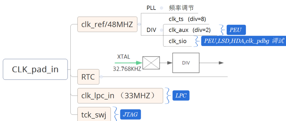
图 4.1 芯片视角时钟域结构
