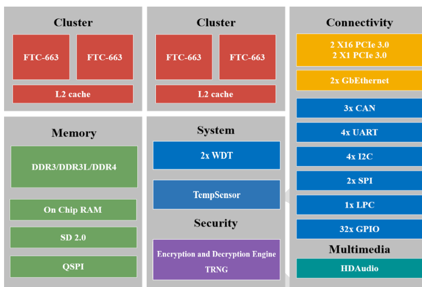
图 1.1 FT-2000/4 功能框图
