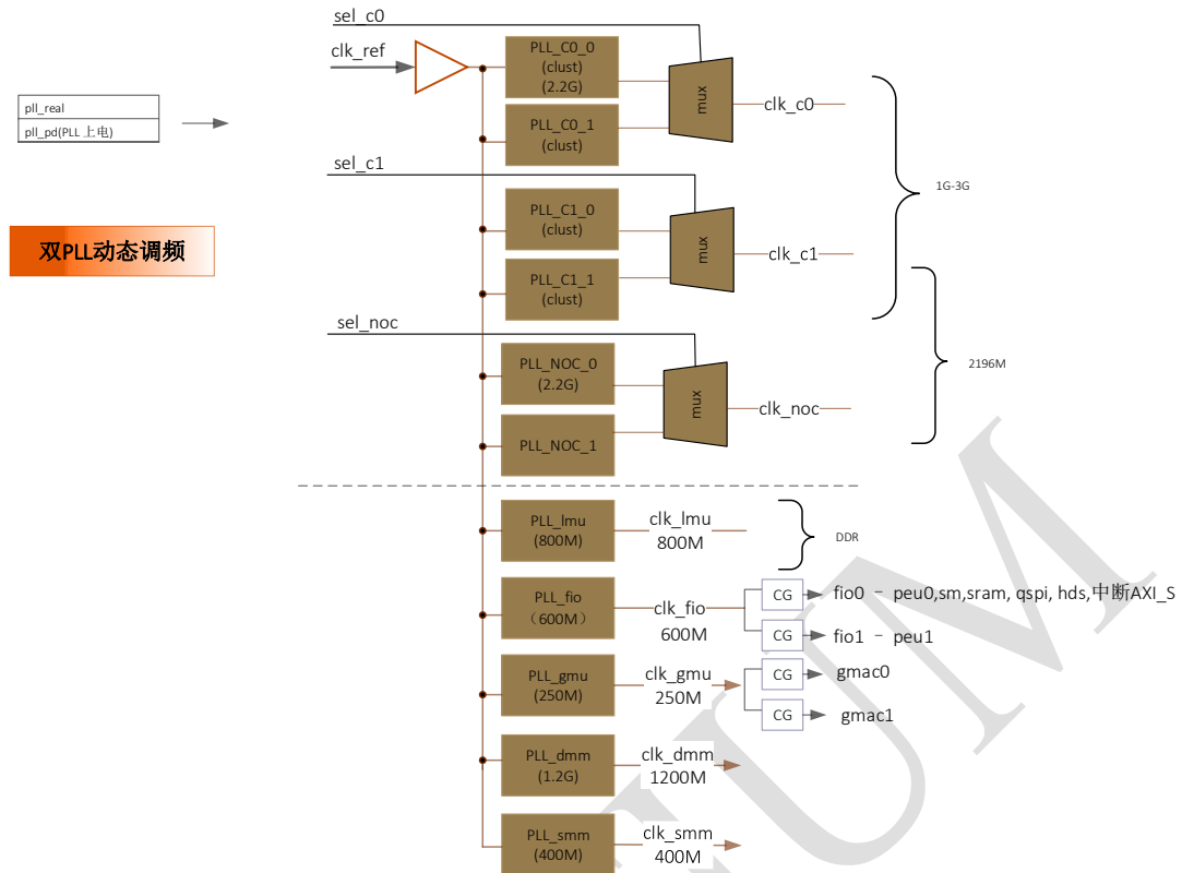
图 4.2 高频时钟域结构
