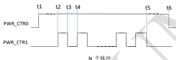
图 5.6 时序图
