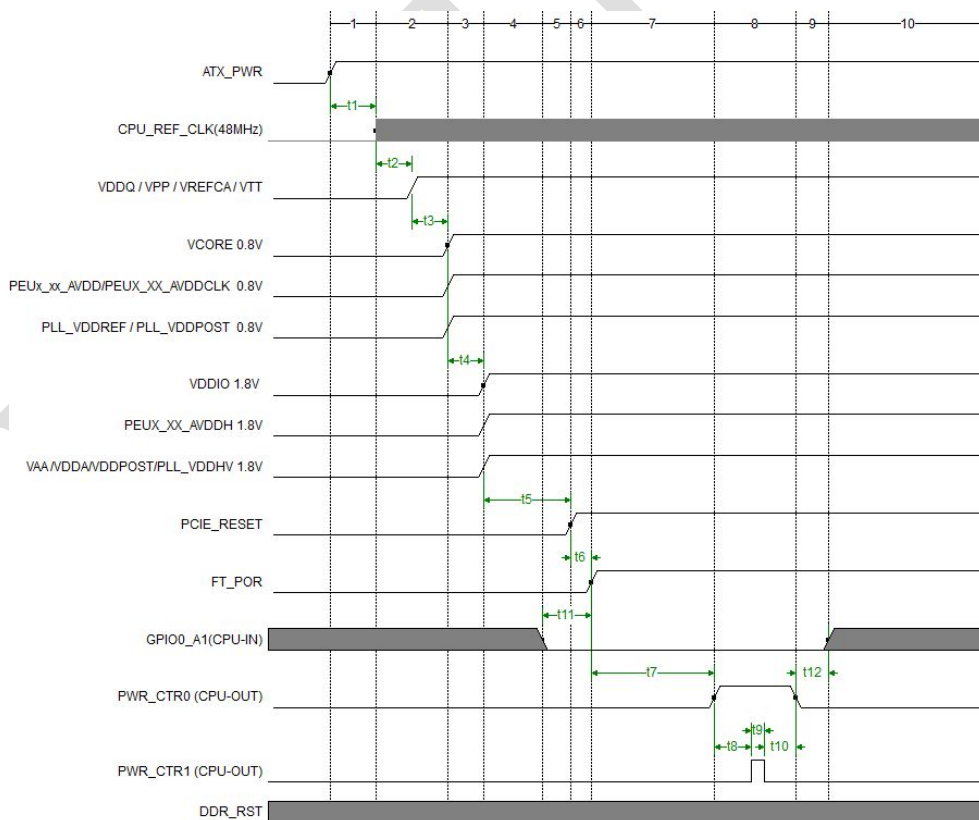
图 5.1 S4/S5→S0 开机时序图
