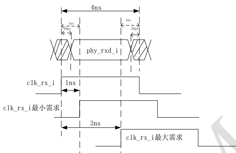
图 2.9 RX 数据端口采样时序图
